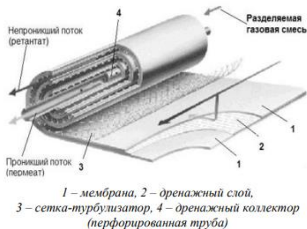
Рис. 2 - Рулонный модуль
